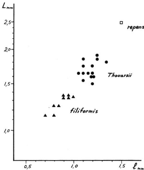
Fig. 2. — Dimensions des akènes mûrs d' Actinoschænus (coordonnées semi-logarithmiques).
